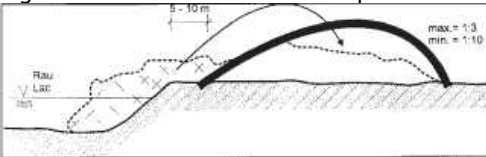
Figura 1.11 - Depozite de deșuri amplasate pe malul apei
