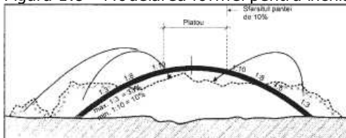
Figura 1.9 Vedere laterală a depozitului
